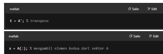
Gambar 2. Operasi Transpose dan Indeksasi Elemen
