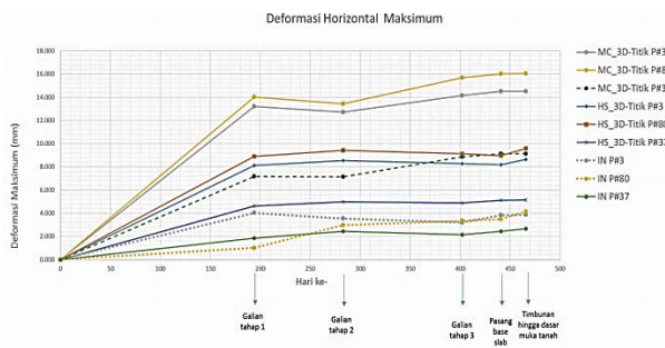
Gambar 8. Deformasi Horizontal Maksimum
