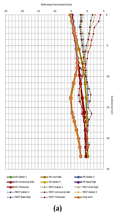
Model Hardening Soil di Titik P#37
