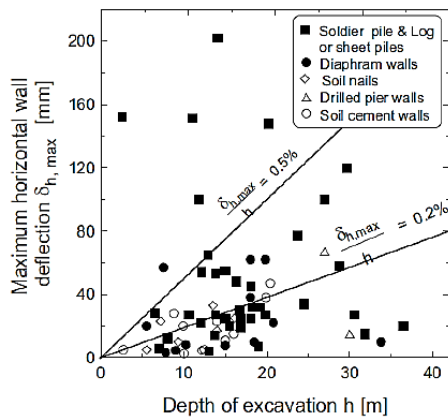
Gambar 1. Pengamatan Defleksi Horizontal Maksimum Dinding Untuk Tipe-Tipe Dinding Pada Tanah Lempung Kaku (Stiff Clay), Tanah Residual, Dan Pasir (Clough Et Al, 1990)
