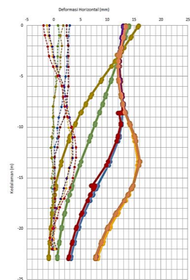
Model Mohr Coulomb di Titik P#80
