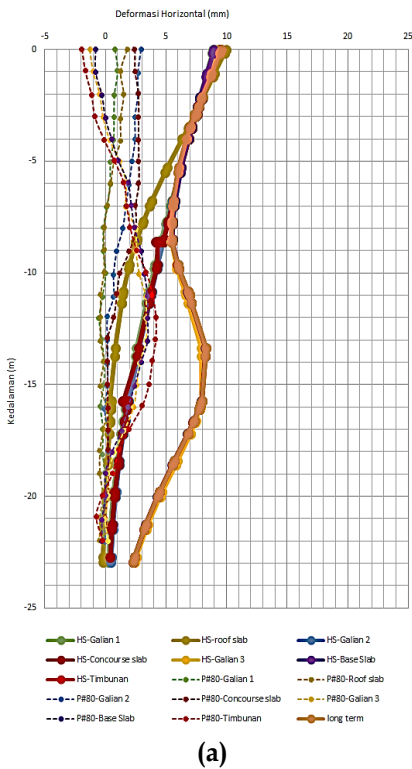
Model Hardening Soil di Titik P#80
