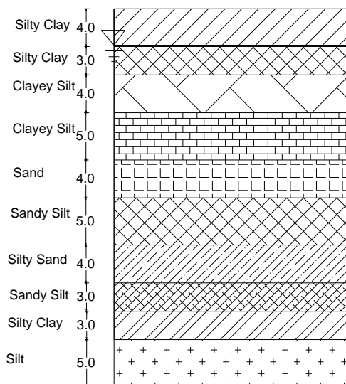
Gambar 2. Profil Tanah Yang Mewakili
