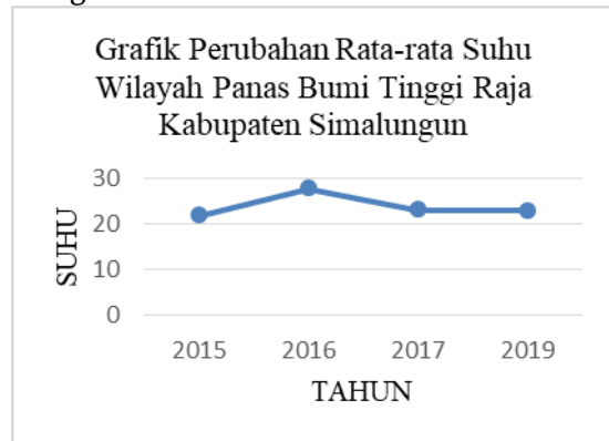
Gambar 3. Grafik Perubahan Rata-Rata suhu Wilayah Panas Bumi Tinggi Raja Kabupaten Simalungun
