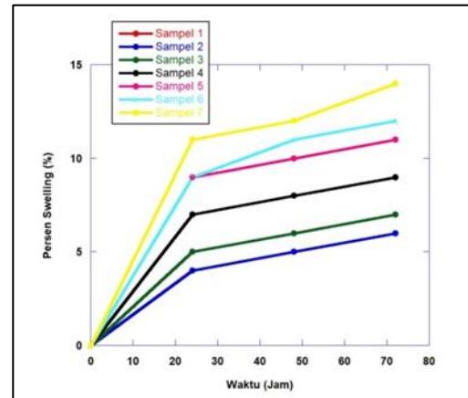
Gambar 3. Hubungan Komposisi terhadap % Swelling
