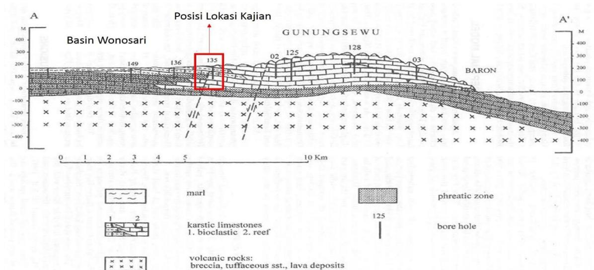
Gambar 2. Lokasi Luweng Belimbing Menempati Peralihan antara Basing Wonosari dan Karst Gunungsewu (Notosiswoyo dan Kusumayudha, 1998 dengan Modifikasi)
