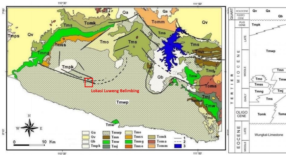
Gambar 3. Lokasi Luweng Belimbing secara Geologi Regional (Modifikasi dari Haryono et al, 2017)
