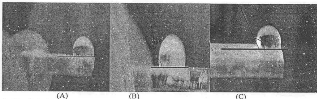
Gambar 3; Sudut kontak antara kaca dengan air pada sampel yang dilapisi \text{TiO}_2 dengan variasi suhu pembakaran (A) suhu 110^\circ\text{C} , (B) suhu 150^\circ\text{C} , (C) suhu 200^\circ\text{C}
