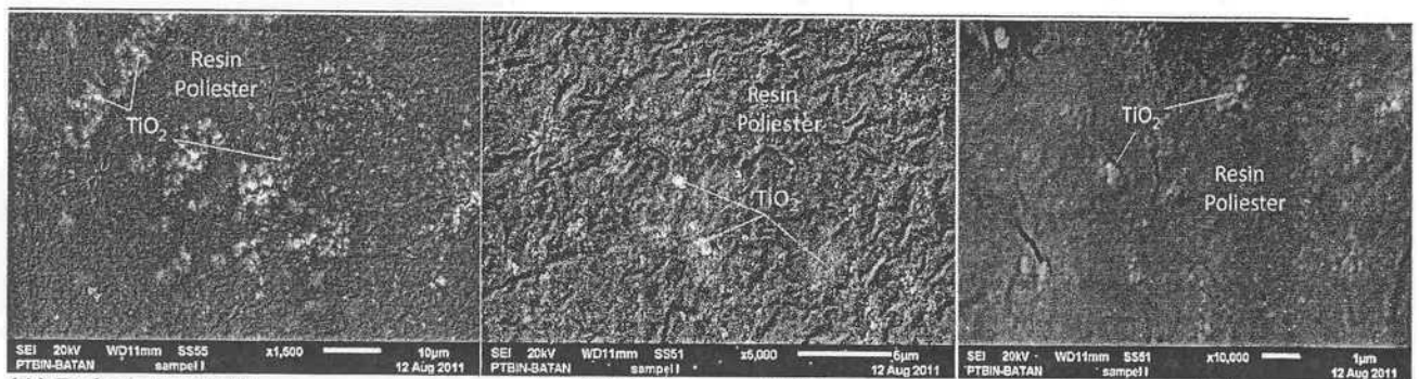
Gambar 9. Thin Film TiO 2 pada logam
