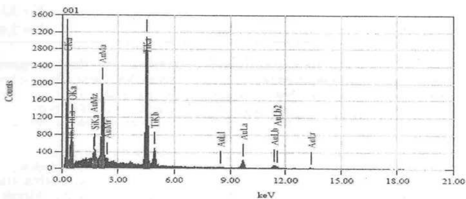
Gambar 10. Analisis elementer sample I Thin Film TiO 2 pada besi
