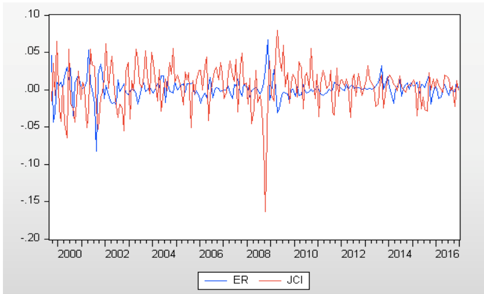
Gambar 1. Pertumbuhan Nilai Tukar IDR/US$ (ER) dan Pertumbuhan IHSIG (JCI).
