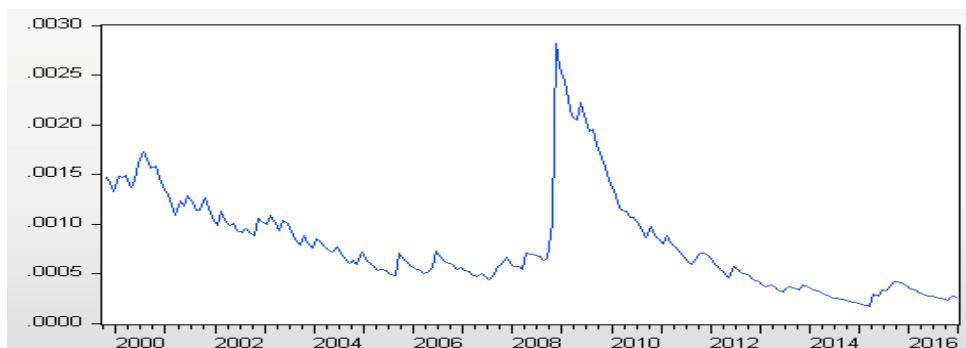
Gambar 5. Volatilitas Antar Waktu dari JCI (VJCI)
