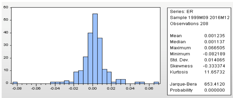
Gambar 2. Statistik Deskriptif Pertumbuhan Nilai Tukar Rupiah atas US Dollar (ER).
