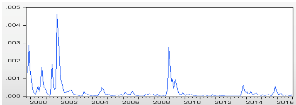
Gambar 4. Volatilitas Antar Waktu dari ER (VER)
