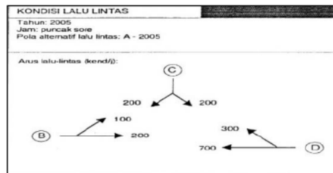
Gambar 2. Contoh sketsa arus lalu lintas (MKJI, 1997).
