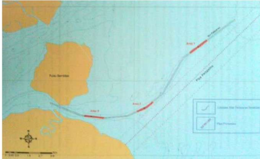
Gambar 4. Tata letak rencana pengerukan.
