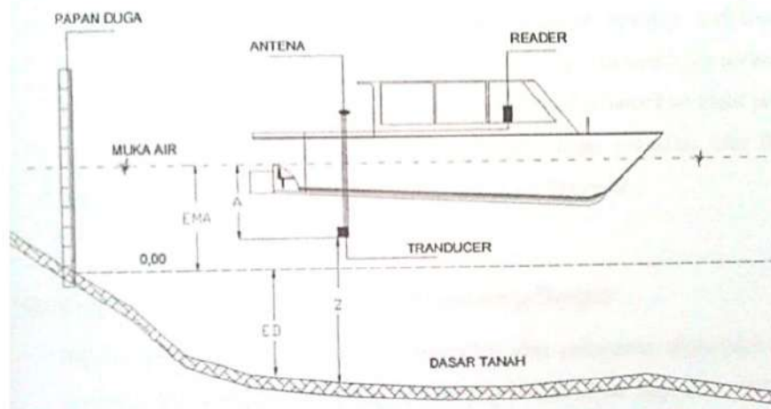
Gambar 3. Penempatan peralatan Echosounder dan GPS Receiver .
