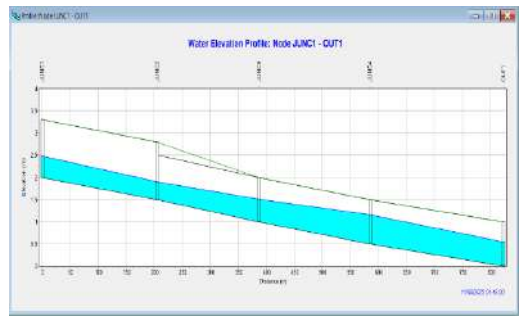
Gambar 7. Profil aliran dari JUN1, JUNC2, JUNC3, JUNC4, dan OUT1 pada selang waktu 1 jam 15 menit (air tidak mengalami peluapan)
