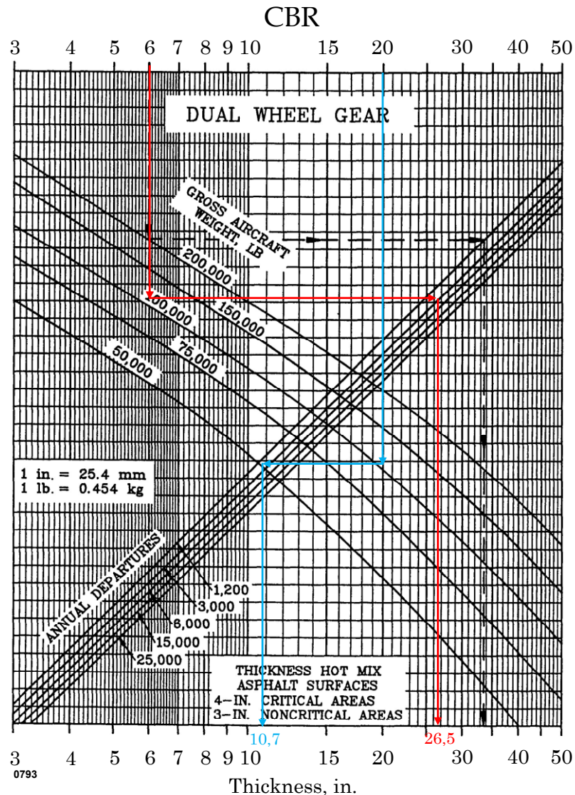
Gambar 2. Penentuan tebal perkerasan total (garis merah) dan lapisan subbase (garis biru) menggunakan metode FAA.
