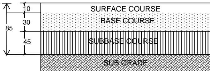
Gambar 4. Tebal Tiap Lapisan Perkerasan pada saat Pelaksanaan.
